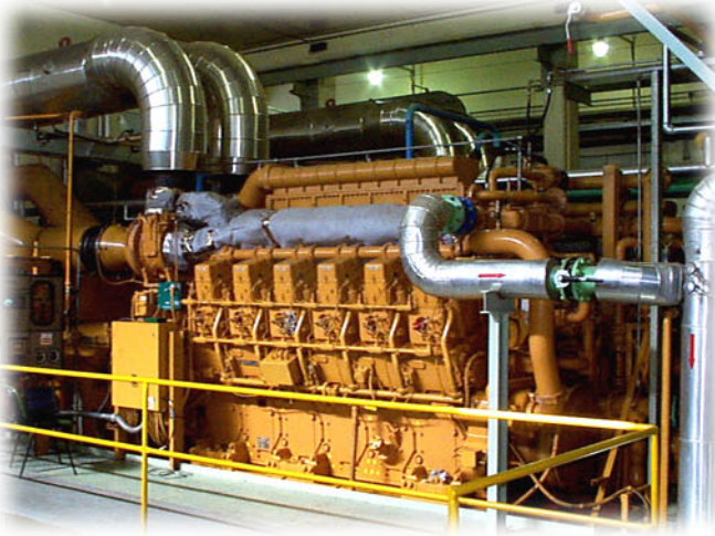
Motor CAT® 3616 en Mercedes, Argentina para Dupont generando 7 MW y usando gas como combustible.
