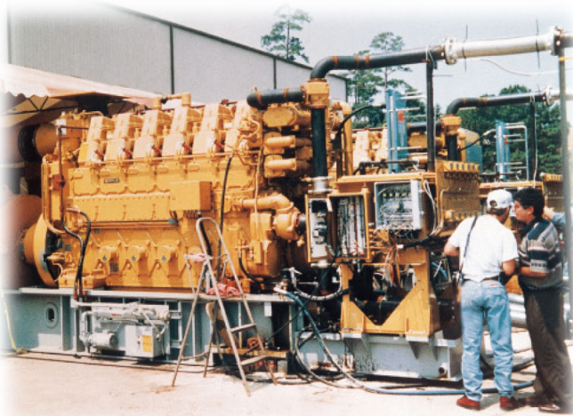
Detalle de generador de energía para campos de perforación, Colombia. Cliente: Agrosy. Cuenta con dos motores CAT® 3606 acoplados a generadores Kato. Los motores usan crudo como combustible.
