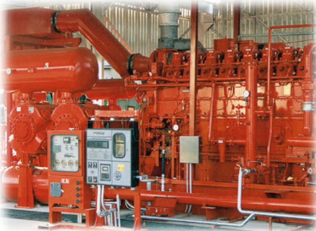
Estación de compresión de gas en Provincia, Colombia con cuatro paquetes de compresión conducidos por motores G3608 de CAT®.
