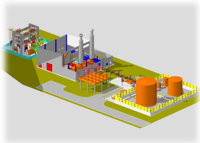
Concepto de diseño de la planta de energía de Caldera que consiste en dos motores 12CM32 que generan 11.2 MW.
